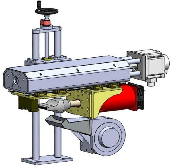
1.2 Kaynak istasyonu
