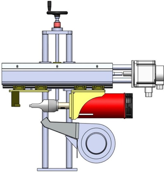
1.3 Kaynak istasyonu
